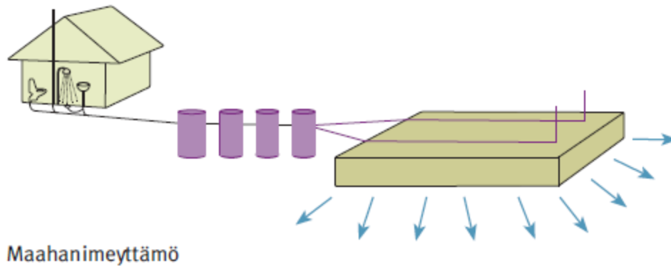
Kuva 2. Maahan imeytyksen periaatekuva
